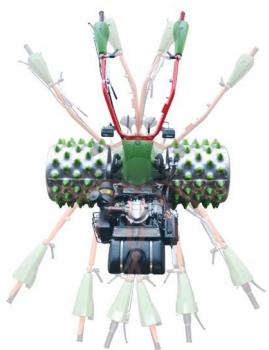
Schwenk- und drehbarer Holm
